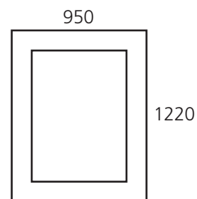
Cadre VERTIZ , en pierre de Brétignac, équipé du foyer DECOSTEEL 4080.
