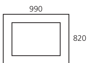
Cadre QUADRO , en pierre de Brétignac, équipé du foyer DECOSTEEL 4090.
